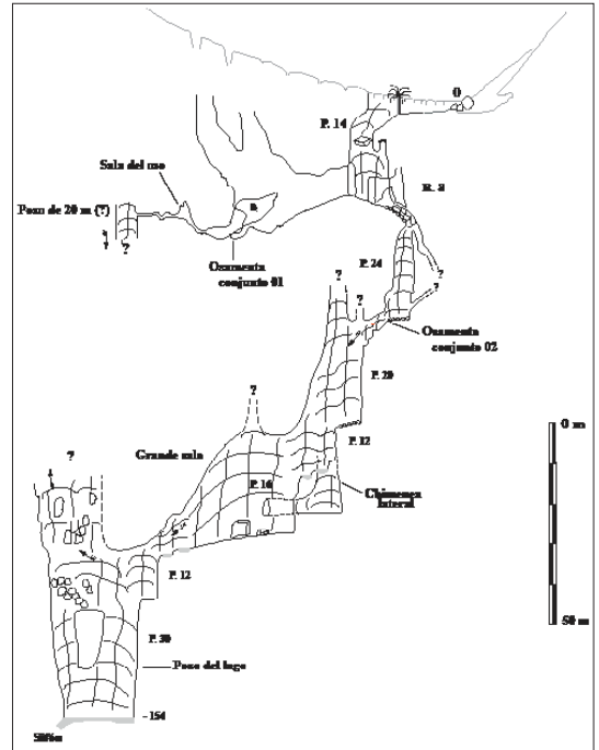
Figura 10 – Corte del tragadero de Chaquil
