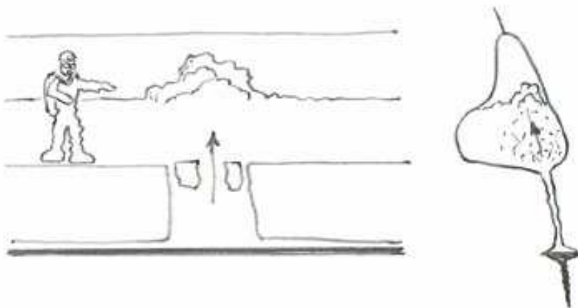
Figure 4 : Reconstitution : coupe longitudinale et section du conduit au droit de la « fissure émissive ».
