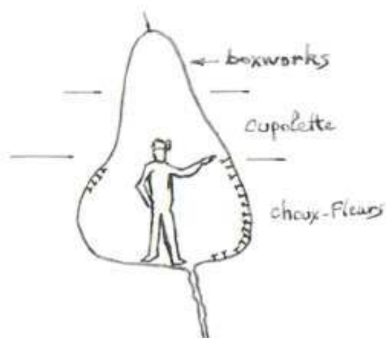
Figure 5 : Répartition des formes pariétales et du concrétionnement dans la galerie de Ceyssole.
