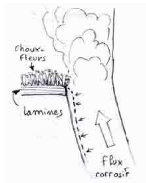
Figure 11 : Coupe schématique du fonctionnement d'une cheminée.
