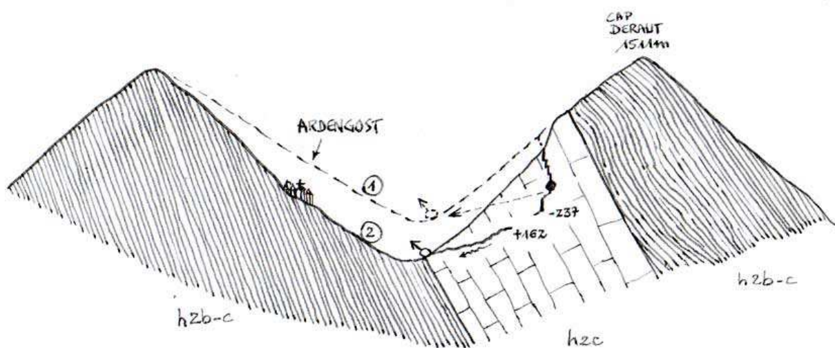
Figure 28 : Coupe schématique de la vallée d'Ardengost et des réseaux Hèche-Charentais.
