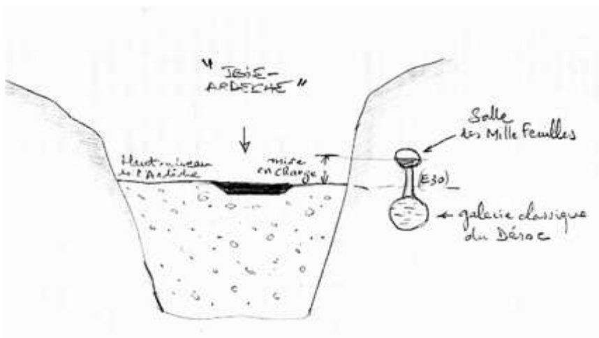
Fig. 7 : Coupe de la grotte du Déroc lors de la formation des lames de la salle des Mille Feuilles.
