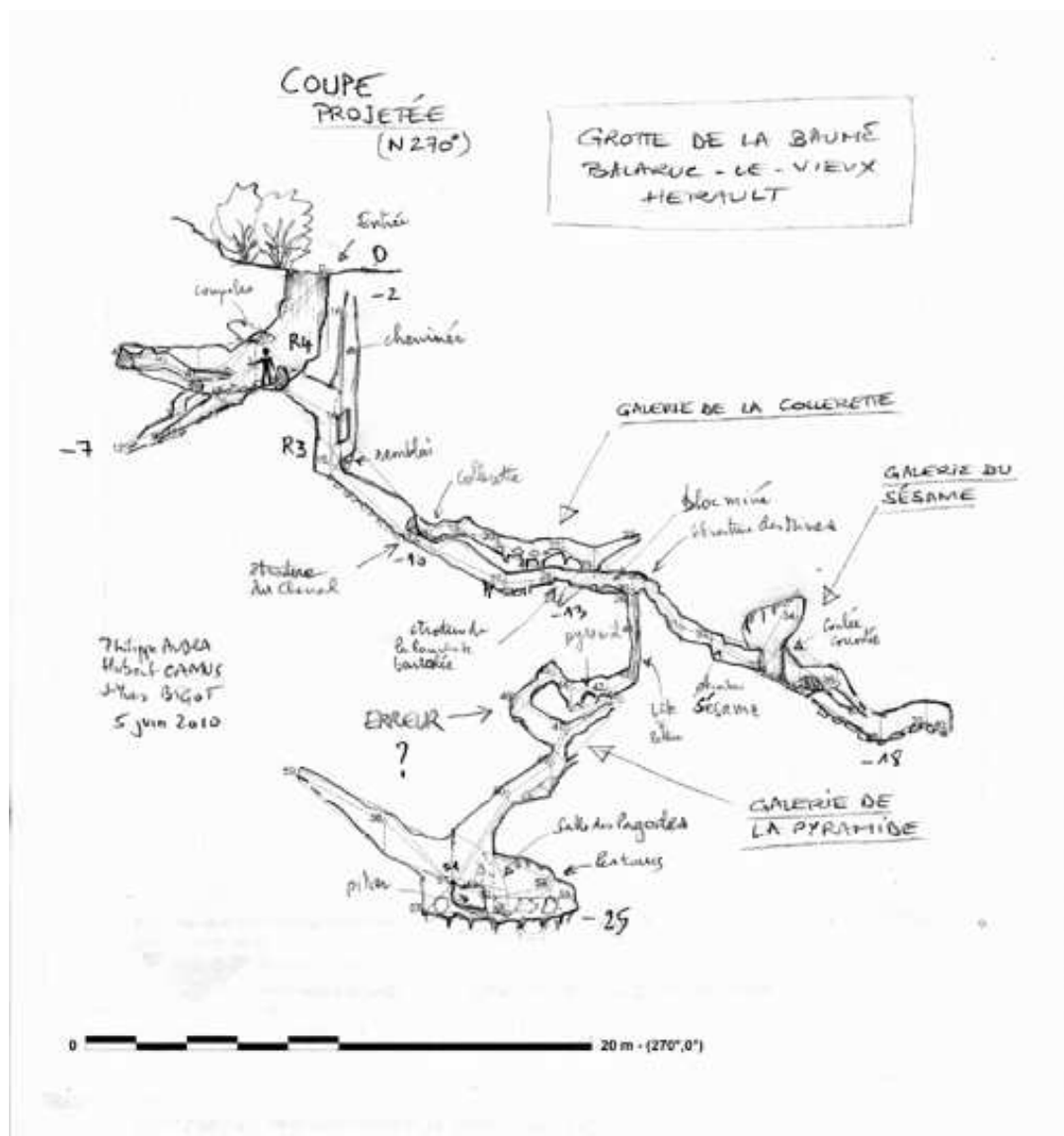
Fig. 12 : Coupe projetée (N270°) de la grotte de la Baume.
