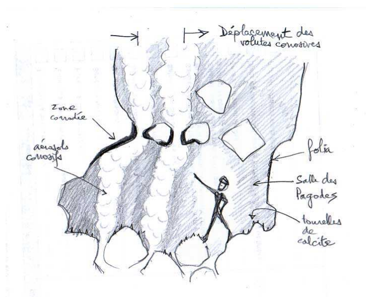
Fig. 12 : Coupe projetée (N270°) de la grotte de la Baume.
