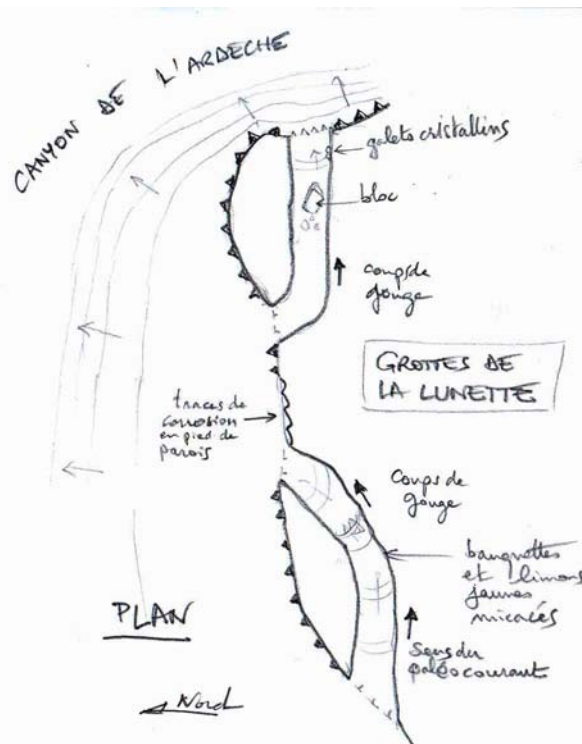
Fig. 9 : Plan schématique des grottes de la Lunette.
