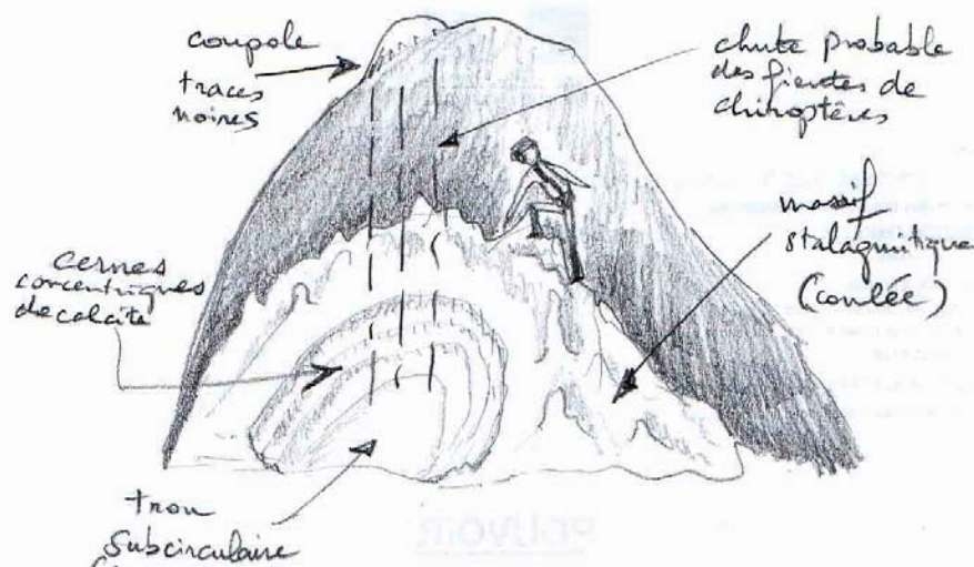
Fig. 6 : Massif stalagmitique affecté par la bio-corrosion.
