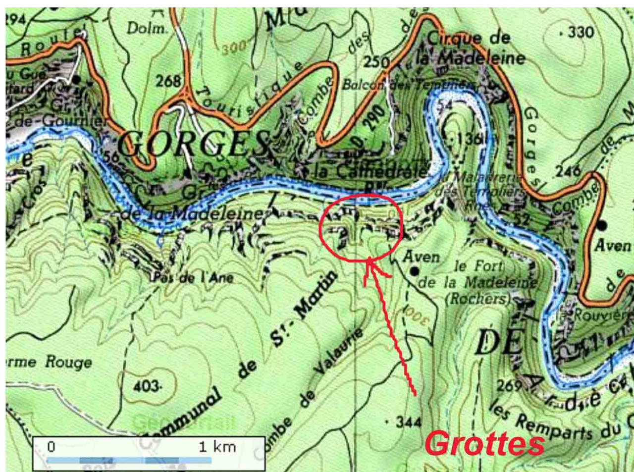
Fig. 3 : Localisation approximative des cavités.
