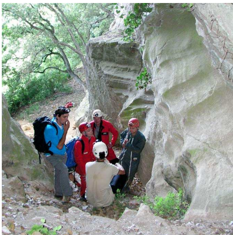
Fig. 2 : Banquettes dans l'entrée de la grotte de la Grosse Marguerite.
