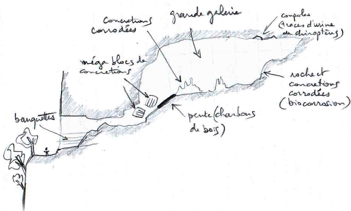
Fig. 4 : Coupe schématique de la grotte de la Grosse Marguerite.
