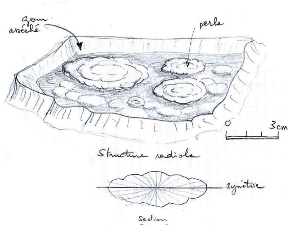
Fig. 7 : Perles des cavernes aplaties dans un gour asséché.
