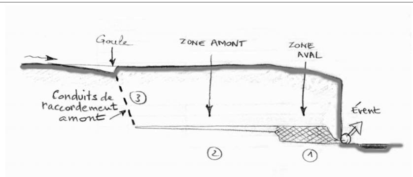
Fig. 7 : Coupe simplifiée représentant les trois zones : 1 : partie aval ; 2 : partie amont ; 3 : conduits de raccordement des puits.
