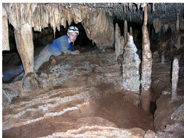
Fig. 3 : Le gour profond et toujours en eau (en bas à droite).
