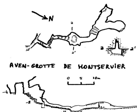
Fig. 7 : Topographie de l'aven-grotte de Montservier extraite du Bull. du Gersam, n° 10, 1990-2000, p. 44.
