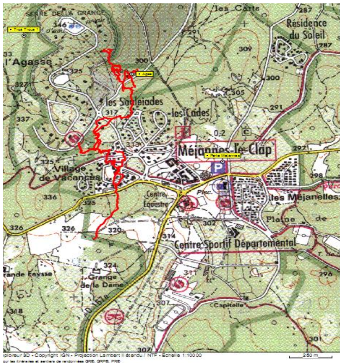
Report sur carte de la topographie de l'aven de L'Agas par Damien Vignoles le 31/05/2014
