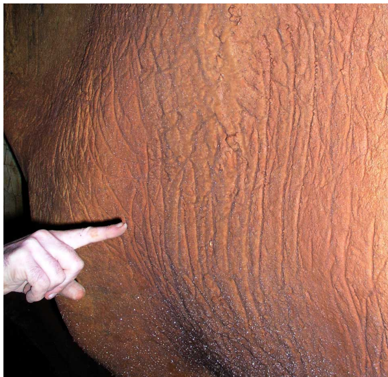
Fig. 1. Griffades (photo du 11-4-2004).
