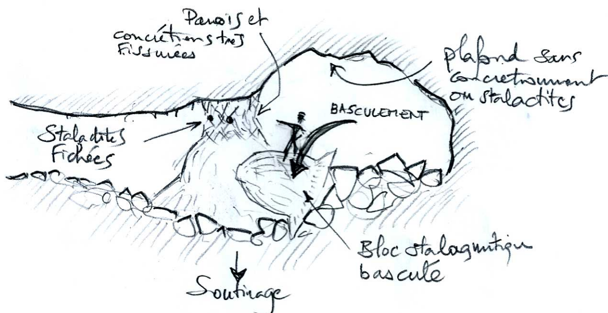
Fig. 12. Coupe de la partie terminale de la grotte où se situent les stalactites fichées.
