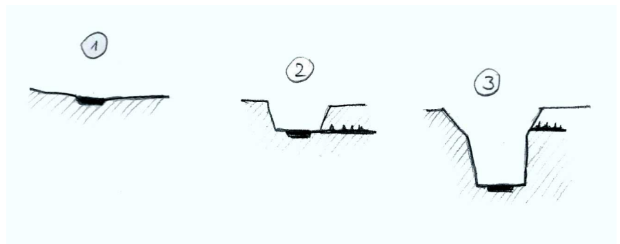
Fig. 5. Différentes phases de creusement des gorges de la Cèze et du plateau de Méjannes. Les vallées et rivières servent de niveau de base aux grottes.
