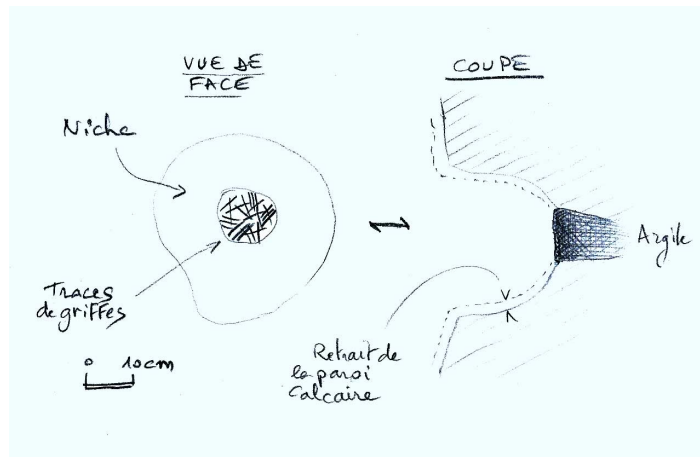
Fig. 7. Coupe et vue de face d'une « niche griffée ».
