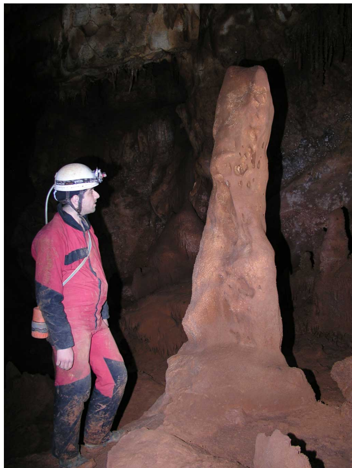
Fig. 3. Grande stalagmite corrodée (photo du 11-4-2004).
