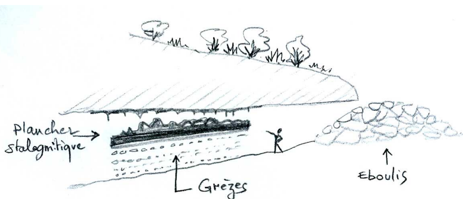
Fig. 6. Coupe schématique de la galerie d'entrée de la grotte du Seigneur.
